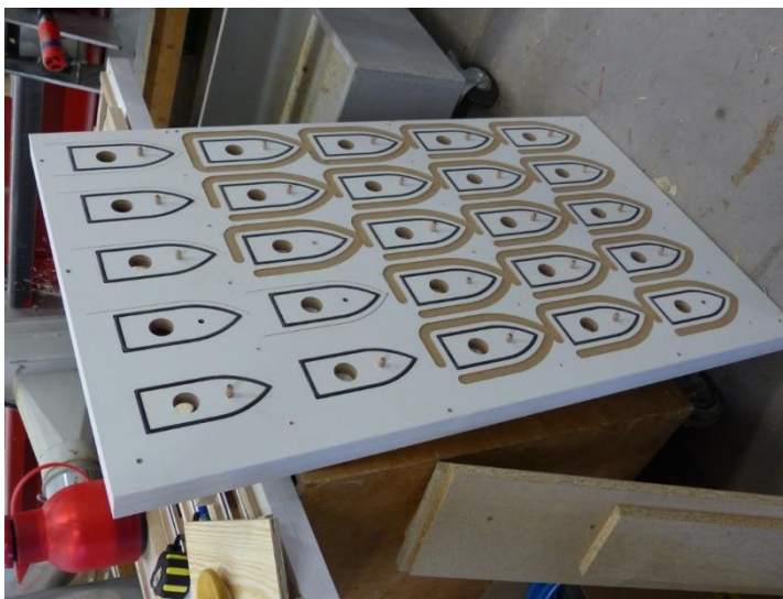
Die Schablonen werden von einem Techniker der Firma Masterwood vor Ort eingefahren.
